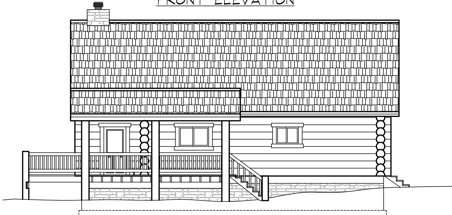
RIGHT ELEVATION
