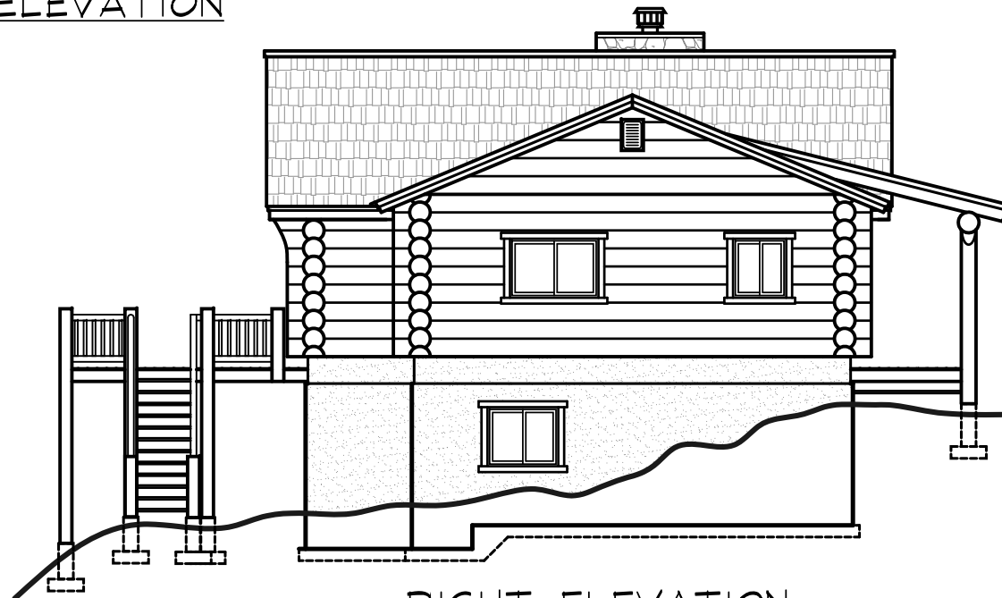
RIGHT ELEVATION
